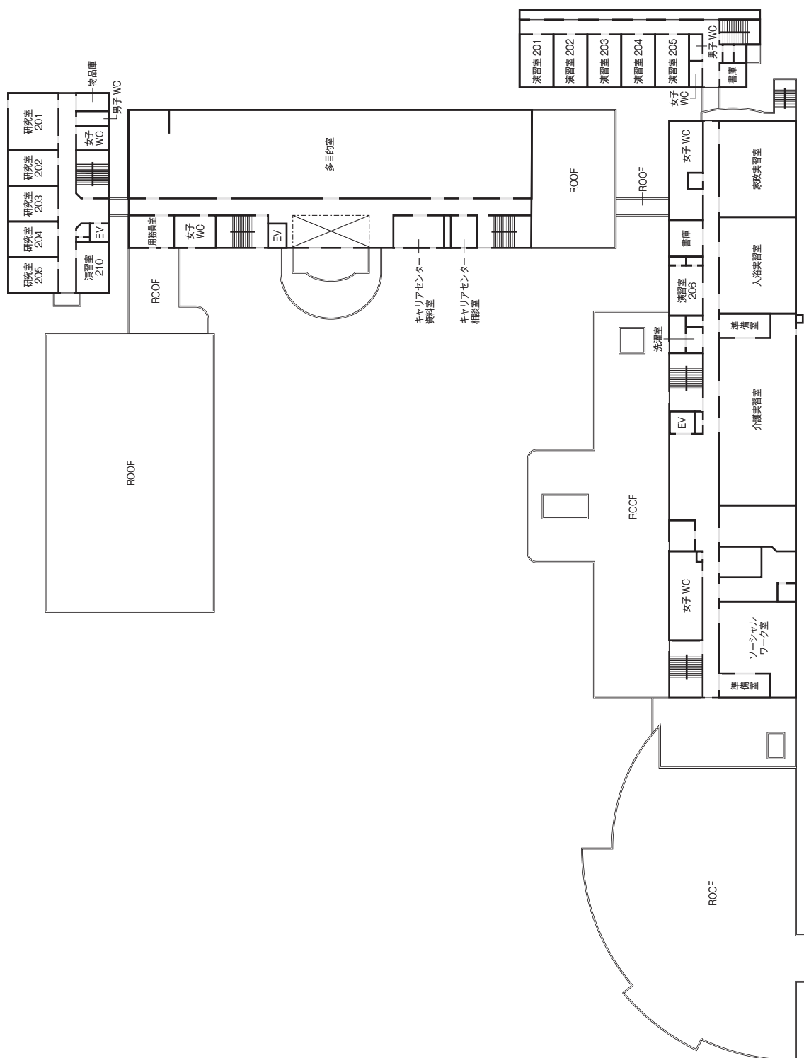
2 階平面図
